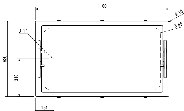
Boven aanzicht
