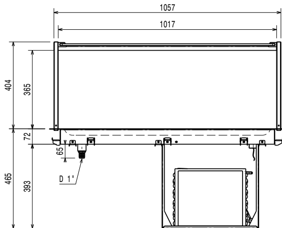
Front aanzicht
